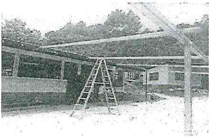
Foto1: Sustitución de cubierta de techo con lámina galvanizada, Tipo de lámina: troquelada Calibre: 26, incluye: fijaciones y sellado en traslapes.
