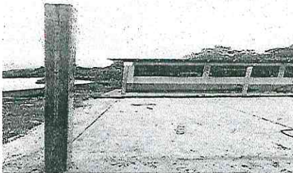
Foto 4: Reparación de losa de concreto para patios, considerando preparación de terreno, armado, nivelación y acabado rustico.
